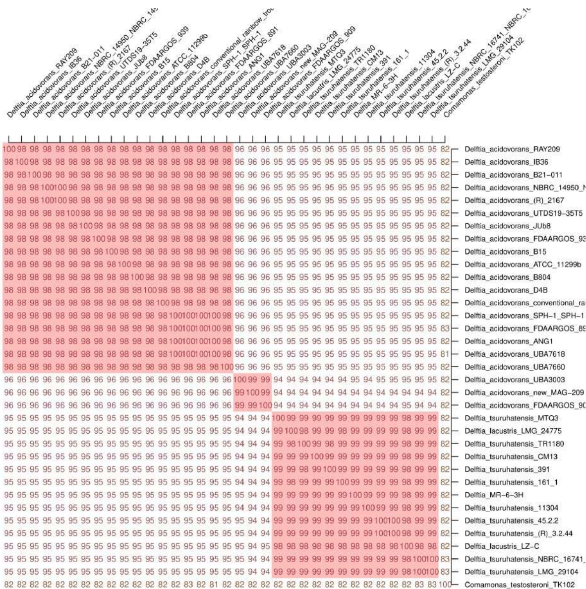
Рисунок 13. Матрица ANI, построенная на сравнении 33 штаммов Delftia spp. с штаммом D. tsuruhatensis MR-6/3H.
