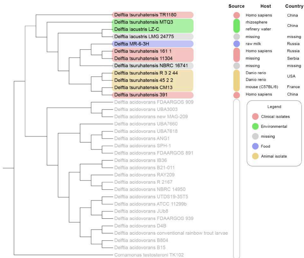
Рисунок 14. Кладограмма, построенная с помощью REALPHY, состоящая из 33 различных штаммов Delftia spp. и штамма D. tsuruhatensis MR-6/3H, основанный на REALPHY: штаммы внутри клады D. tsuruhatensis / D. lacustris отмечены цветом в зависимости от типа источника выделения.
