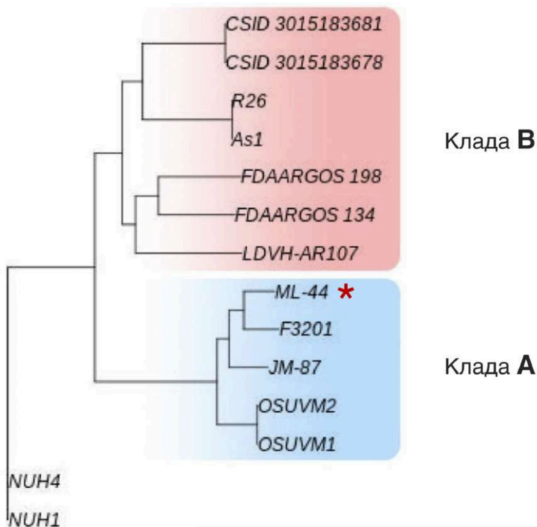
Рисунок 8. Реконструкция кладограммы REALPHY. Штамм ML-44 отмечен бордовой звездочкой.
