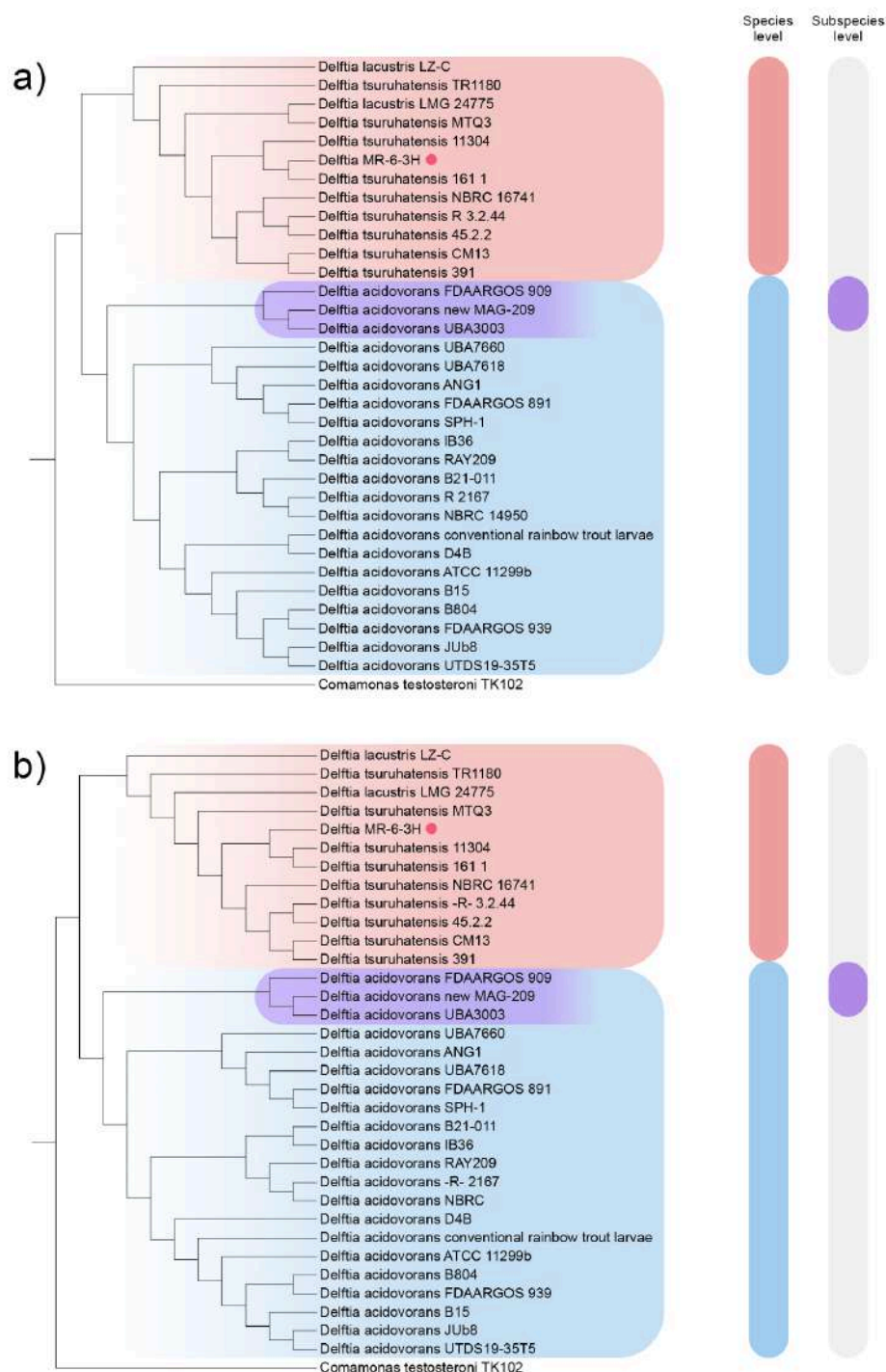
Рисунок 12. Реконструкция кладограмм 33 штаммов Delftia spp. с штаммом D. tsuruhatensis MR-6/3H (отмечен розовым кружком): а) Кладограмма TYGS. б) Кладограмма ANI. Отмечено красным - клада D. tsuruhatensis/lacustris , отмечено синим - клада D. acidovorans , отмечено фиолетовым - предполагаемый подви́д D. acidovorans .
