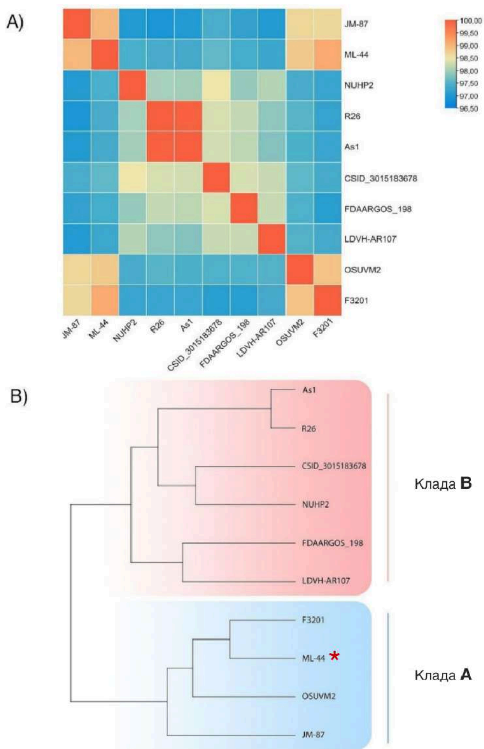
Рисунок 9. Результаты анализа OrthoANI (расчет средненуклеотидной идентичности): (А) Тепловая карта, построенная на значениях ANI между штаммом ML-44 и 9 штаммами E. anopheles ; (В) Кладограмма, реконструированная на основе расчетов OrthoANI. Штамм ML-44 отмечен бордовой звездочкой.
